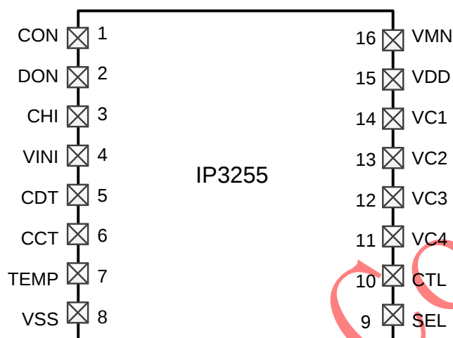
图 1 IP3255 引脚图
