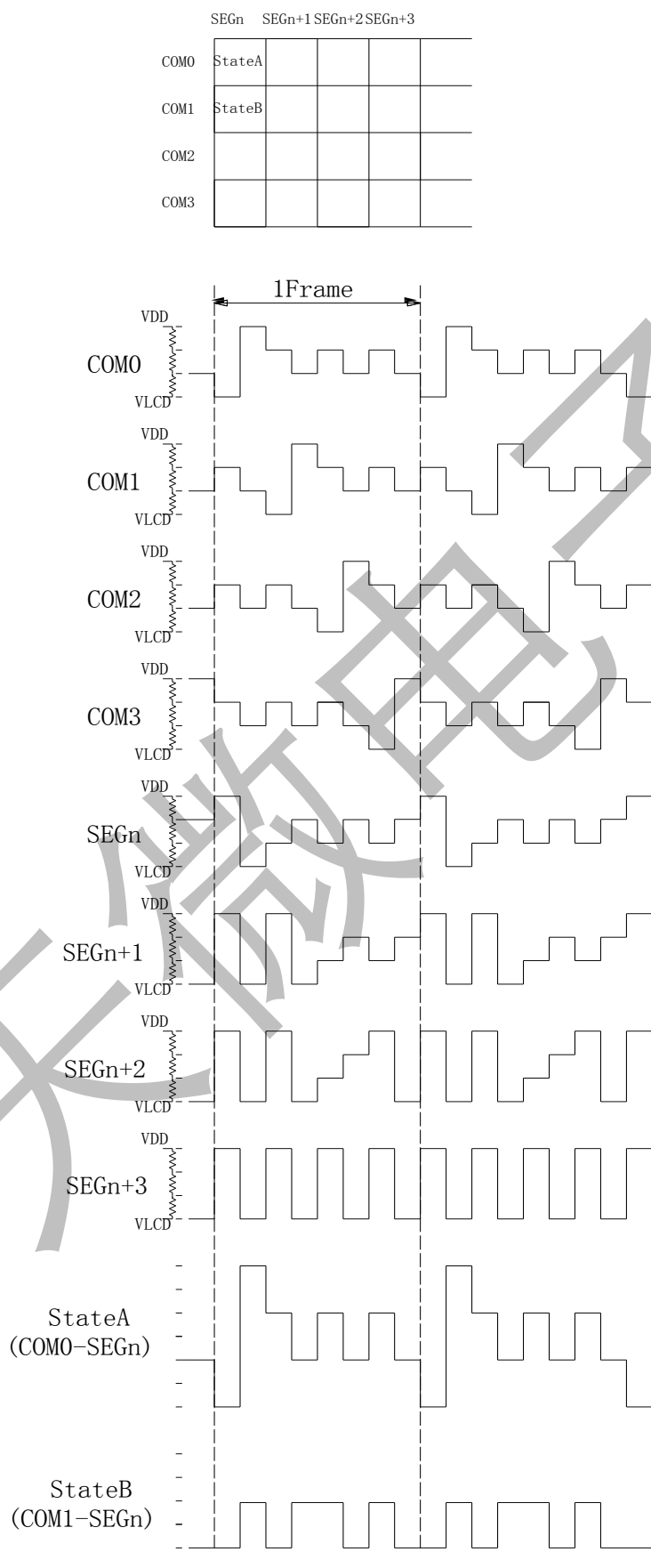
(1) 1/3Bias, Line翻转的液晶驱动波形
