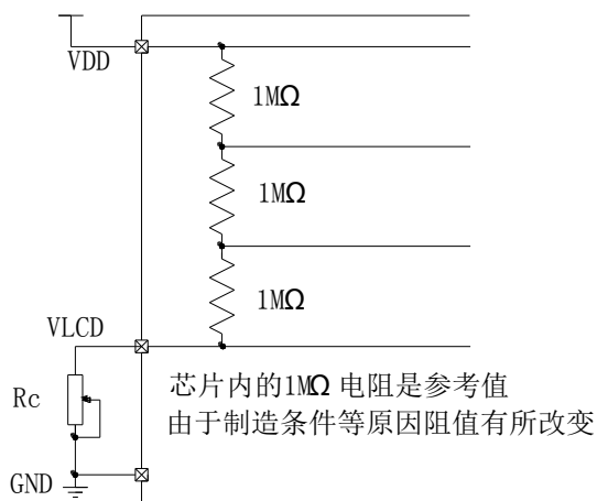
1/3Bias使用对比度调整功能
