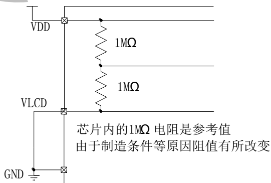
1/2Bias不使用对比度调整功能
