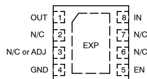
DFN8/DFNW8 3x3 mm (Top View)
