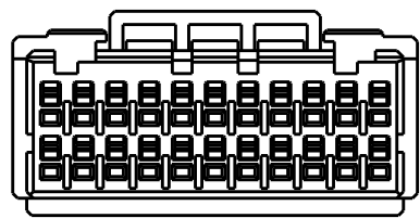
22POS(X-KEY): I-2333134-1
