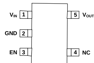
SOT25
