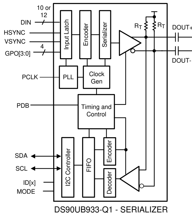
DS90UB933-Q1 - SERIALIZER
